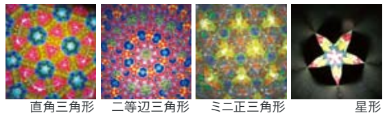
直角三角形
